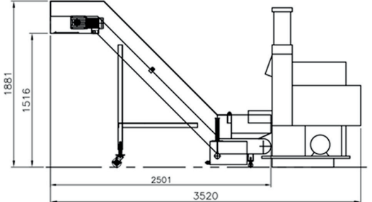
成品傳送機
