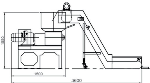
雙軸破碎機
